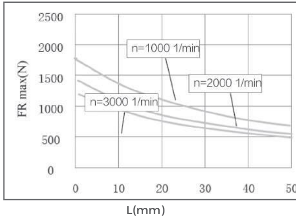
FO=0 N
