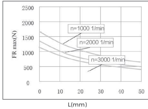
FO=200 N
